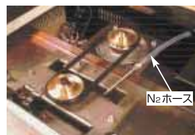
TOP-355APF取付例
